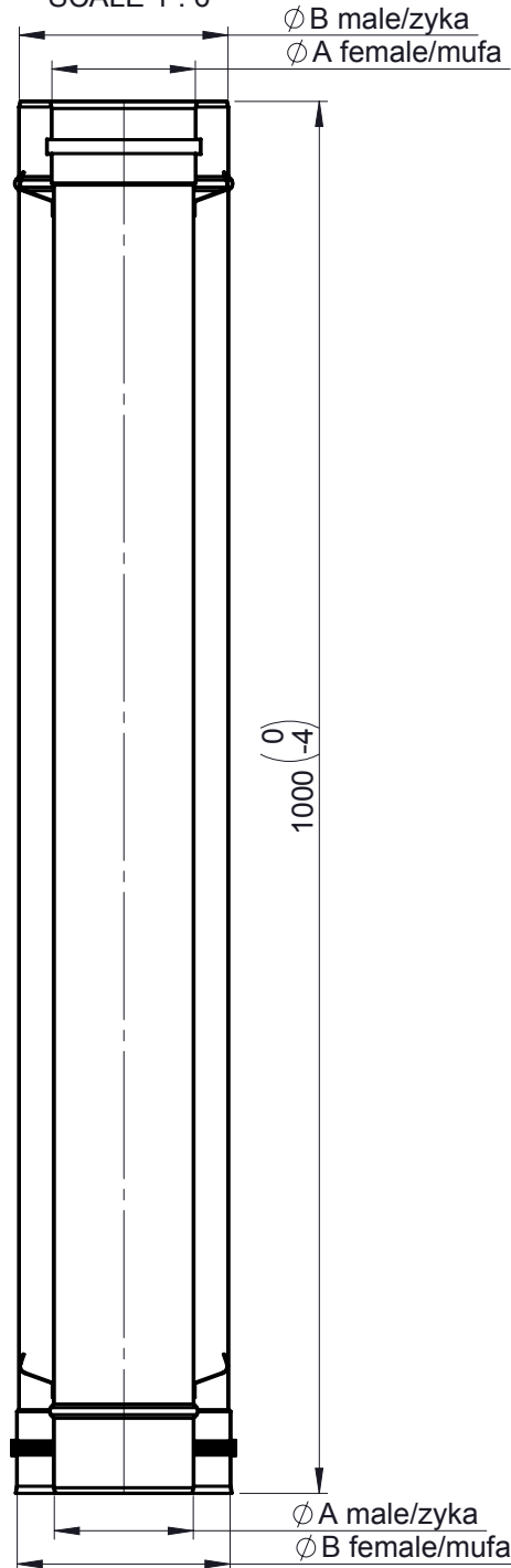
SECTION A-A SCALE 1 : 6
