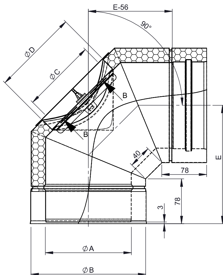
SCHNITT B-B MAßSTAB 1 : 4
