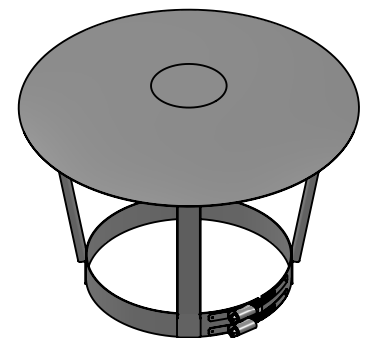
M 1:8 (Ø150)
