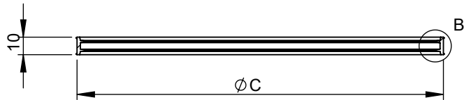
SCHNITT A-A
